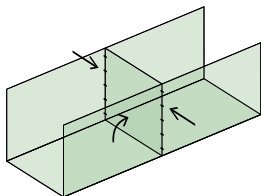
3 Trennwand aufklappen und Längsseiten verbinden (Spiralen oder Klammern)
