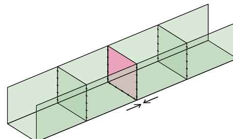
4 Basispaket platzieren und mit Seitenset und nachfolgendem Basispaket verbinden
